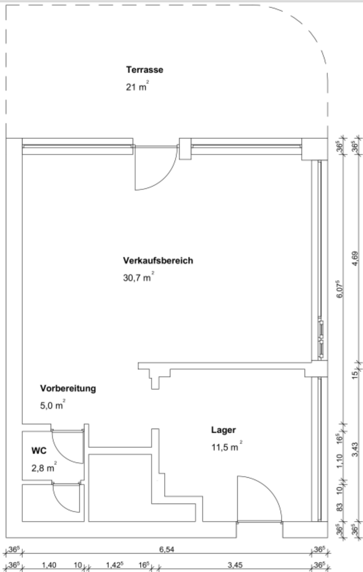
Grundriss Erdgeschoß , Nestroystraße 2, M 1:50
