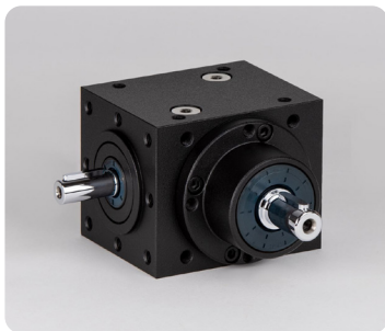
Ritzelwelle am Abtrieb
