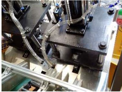
Blick auf die Präge- und Formstation mit Sicherheitsverkleidung
